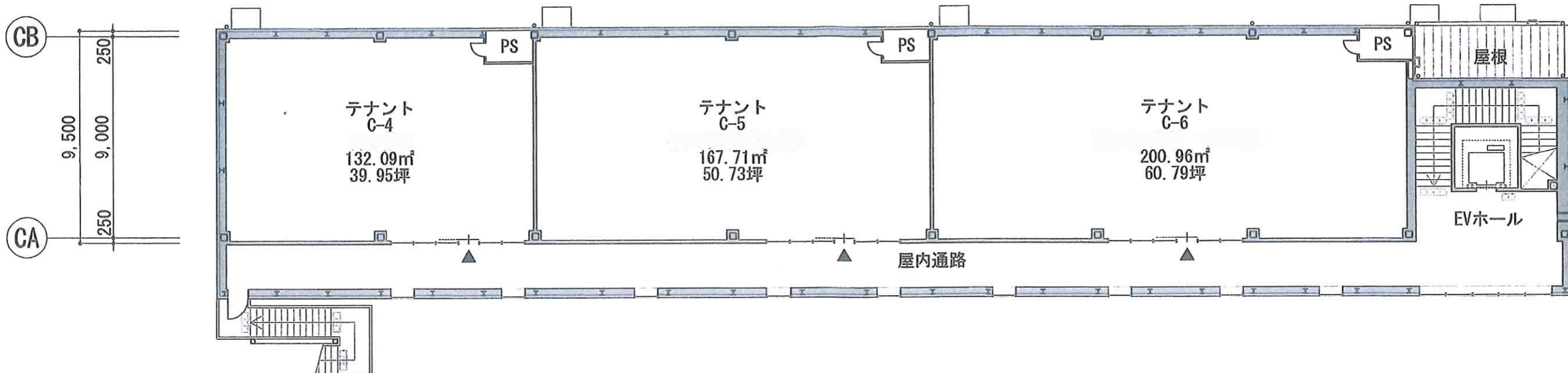
2 階 平 面 図
