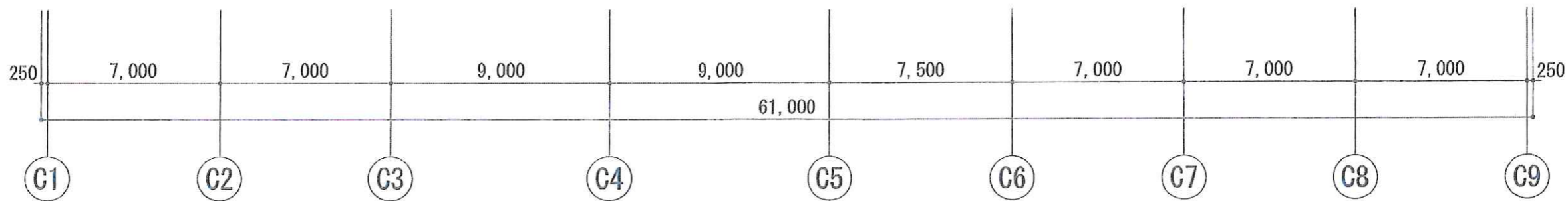
1 階 平 面 図
